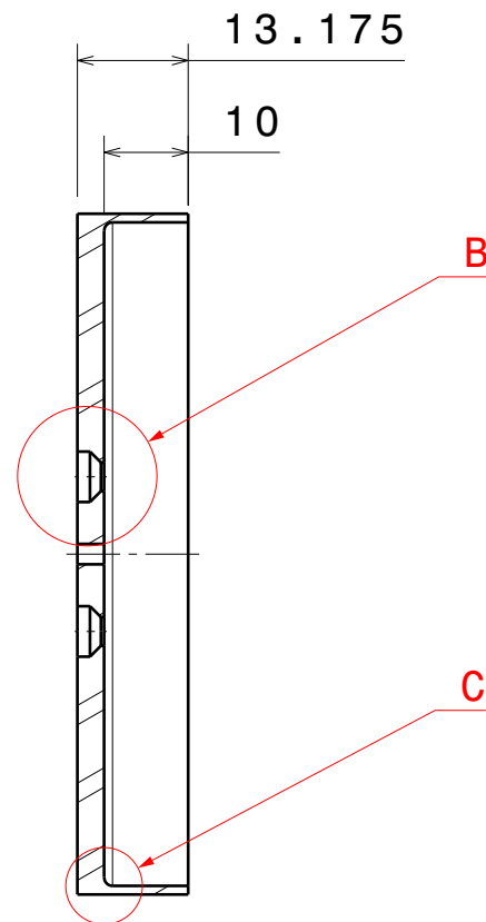
CORTE A-A
